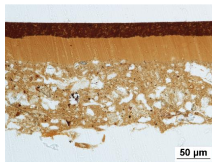
顕微鏡で見た漆塗膜の断面
