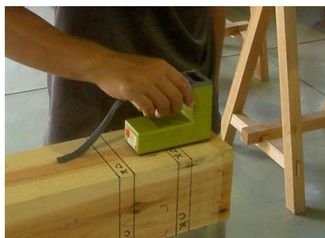
木材の含水率計測状況
